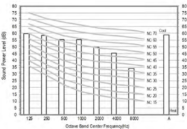
4) CNH364DB (AC036BN4DCH/AA)
