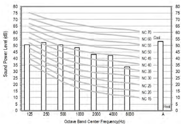
4) CNH364DB (AC036BN4DCH/AA)
