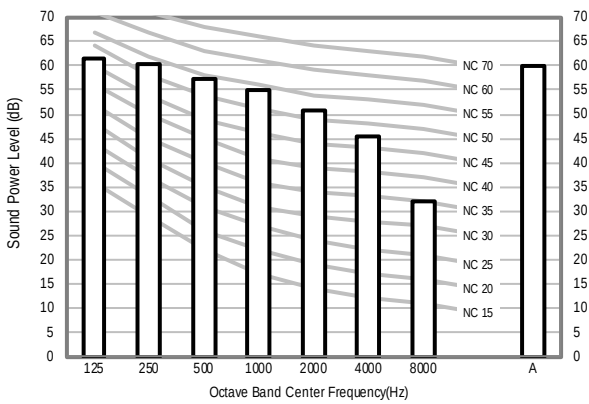
3) CNH30HDB (AC030BNHDCH/AA)
