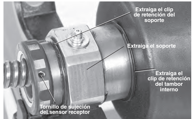
Figure 29 – Extracción del aro de retención y tambor interno
