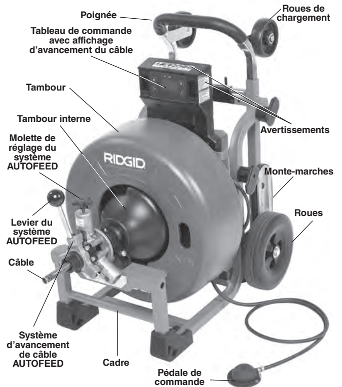
Figure 1A – Dégorgeoir a tambour RIDGID K-4310 FXP
