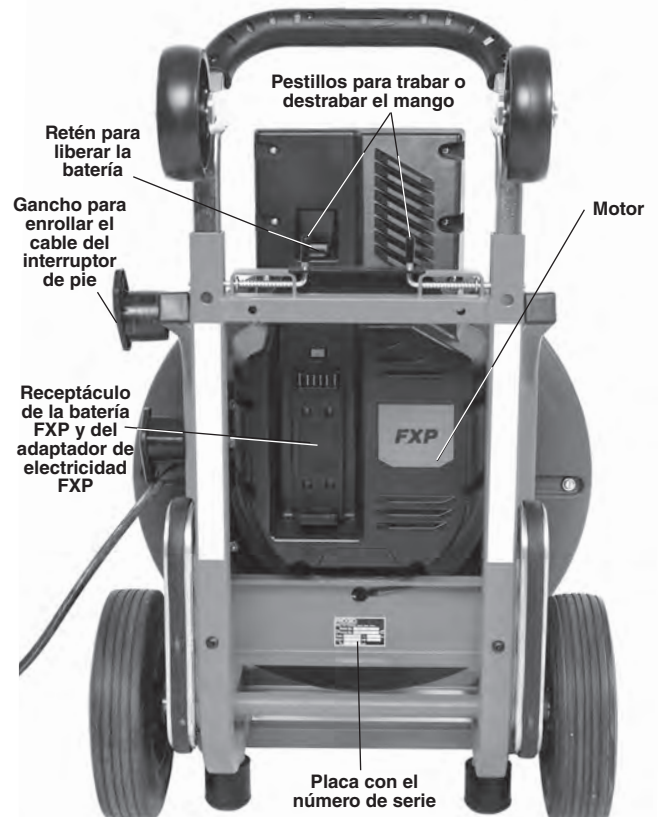
Figura 1 B – Máquina de tambor K-4310 FXP de RIDGID
