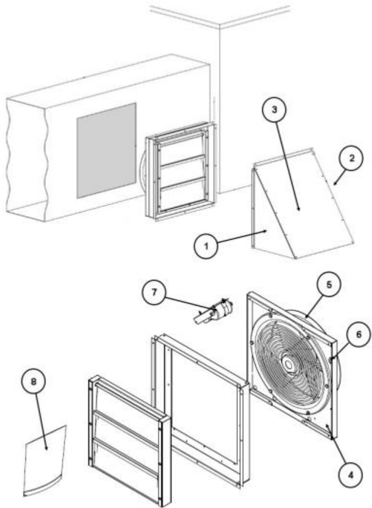
RXRX-CCF03C Assembly
