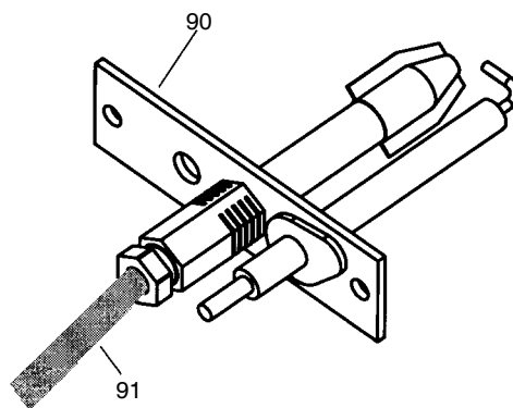
IID LO NOX PILOT
