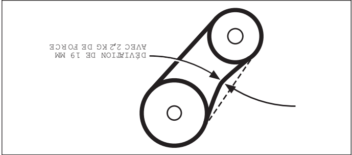
Figure 19.3 - Réglage de tension de la courroie
