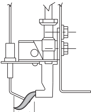
Figure 15.1 - Flamme de veilleuse correcte
