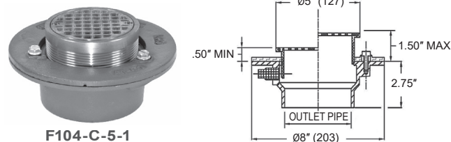
F104-C-5-1
