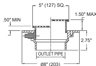
F104-30-S5-1
