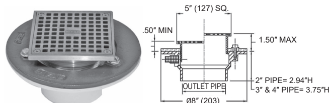
F104-30-C-S5-1
