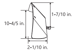
3. Sealplate
