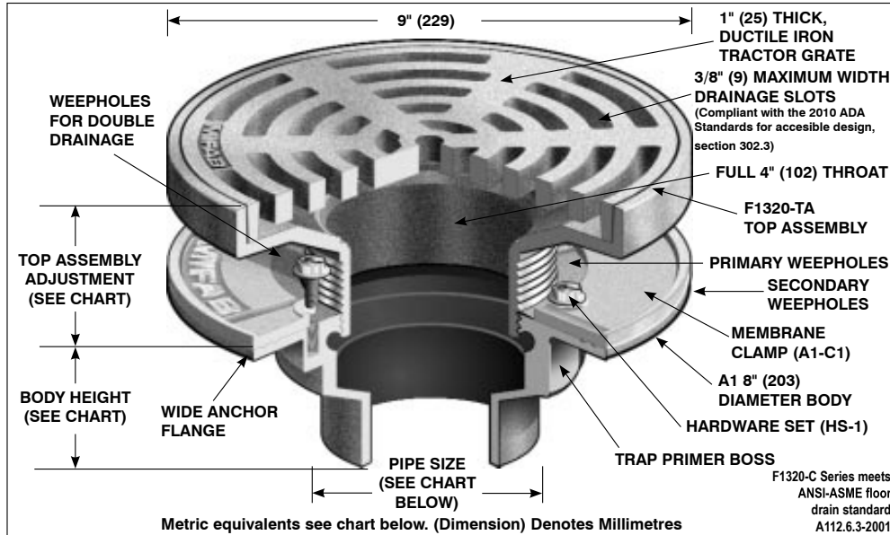
A1 BODY
