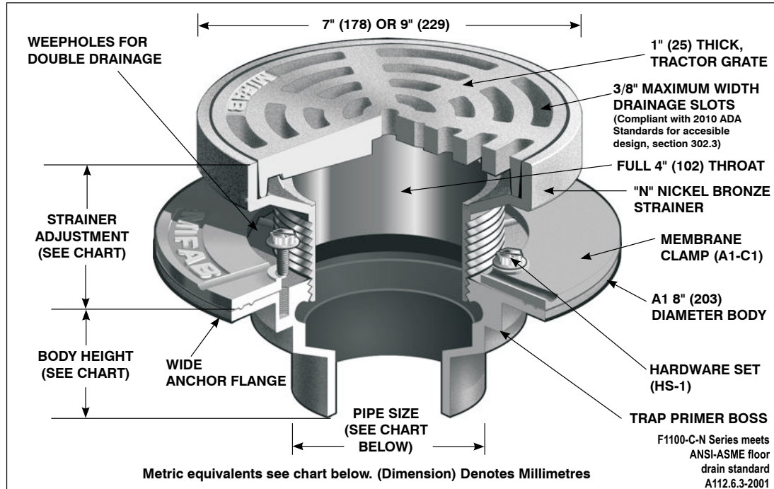
A1 BODY
