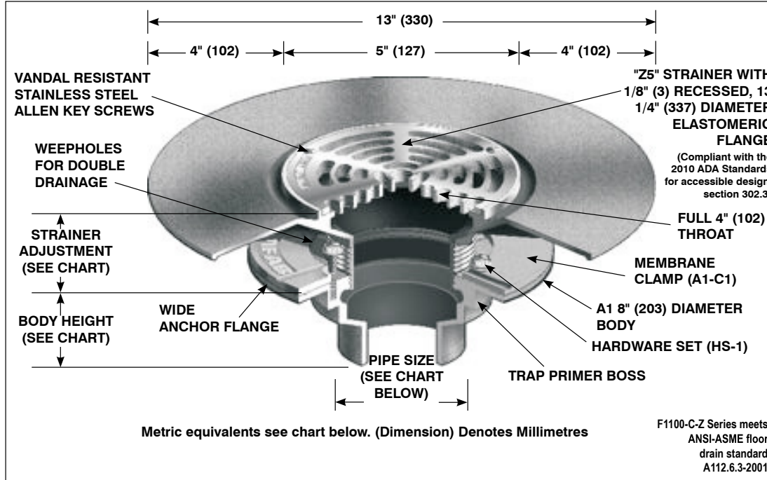
A1 BODY
