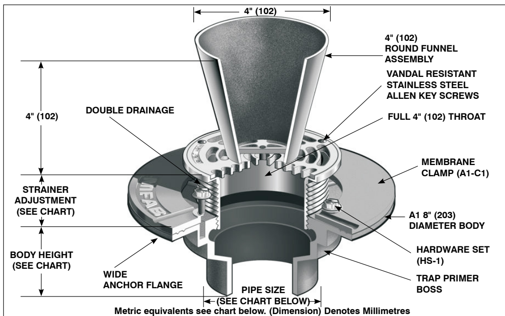
A1 BODY
