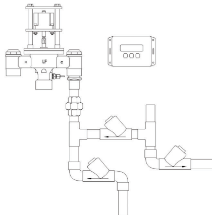
PNV-125-LF-R Simple Recirculation
