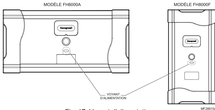
Fig. 17. Voyant d'alimentation.
