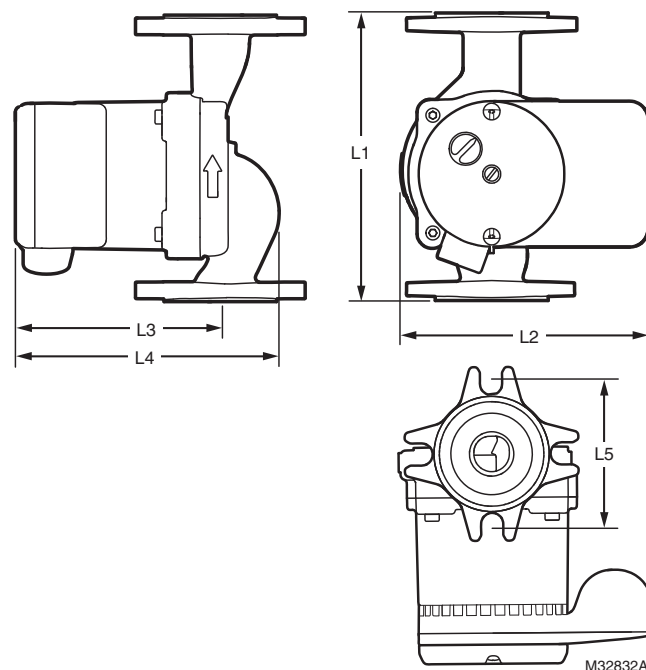
Fig. 1. Dimensiones de la bomba en pulgadas (mm).
