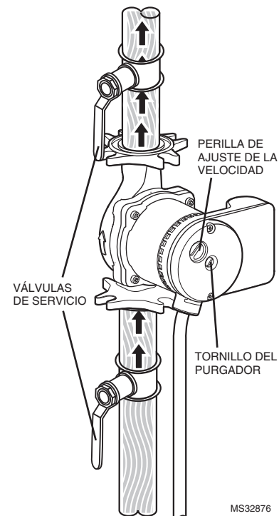
Fig. 9. Purgue el circulador aflojando el tornillo del purgador.
