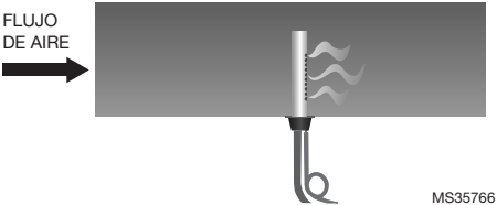
Fig. 10. Distribuidor instalado verticalmente en un conducto horizontal. Esta configuración no se recomienda.
