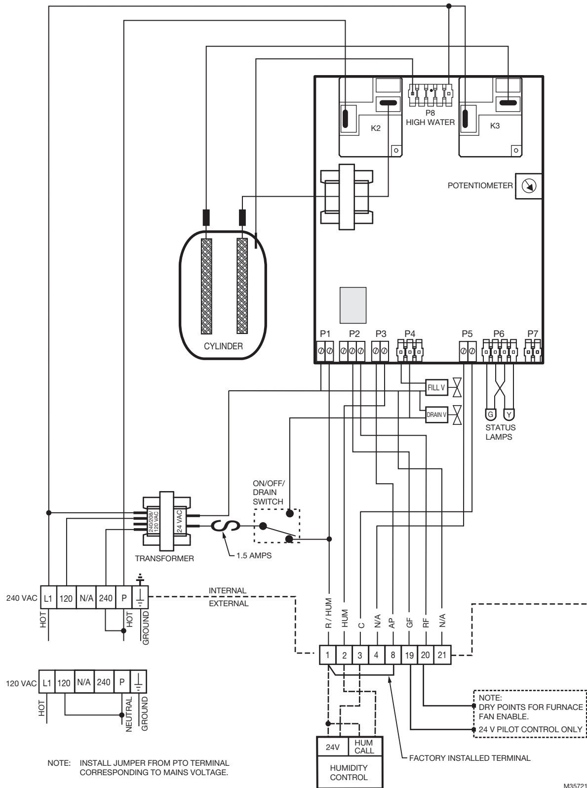
Fig. 26. Wiring diagram.
