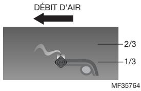
Fig. 8. Distributeur installé horizontalement dans un conduit horizontal.
