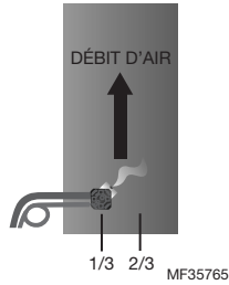
Fig. 9. Distributeur installé horizontalement dans un conduit vertical. Faites tourner le distributeur de 45° pour que la vapeur soit déchargée vers le centre de la gaine, en direction du débit d'air.
