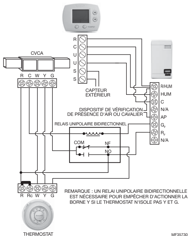
Fig. 18. Câblage de l'humidificateur à vapeur avec un thermostat mécanique.
