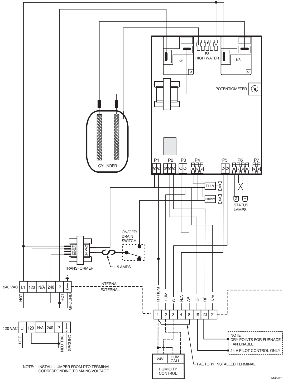
Fig. 4. Wiring diagram.
