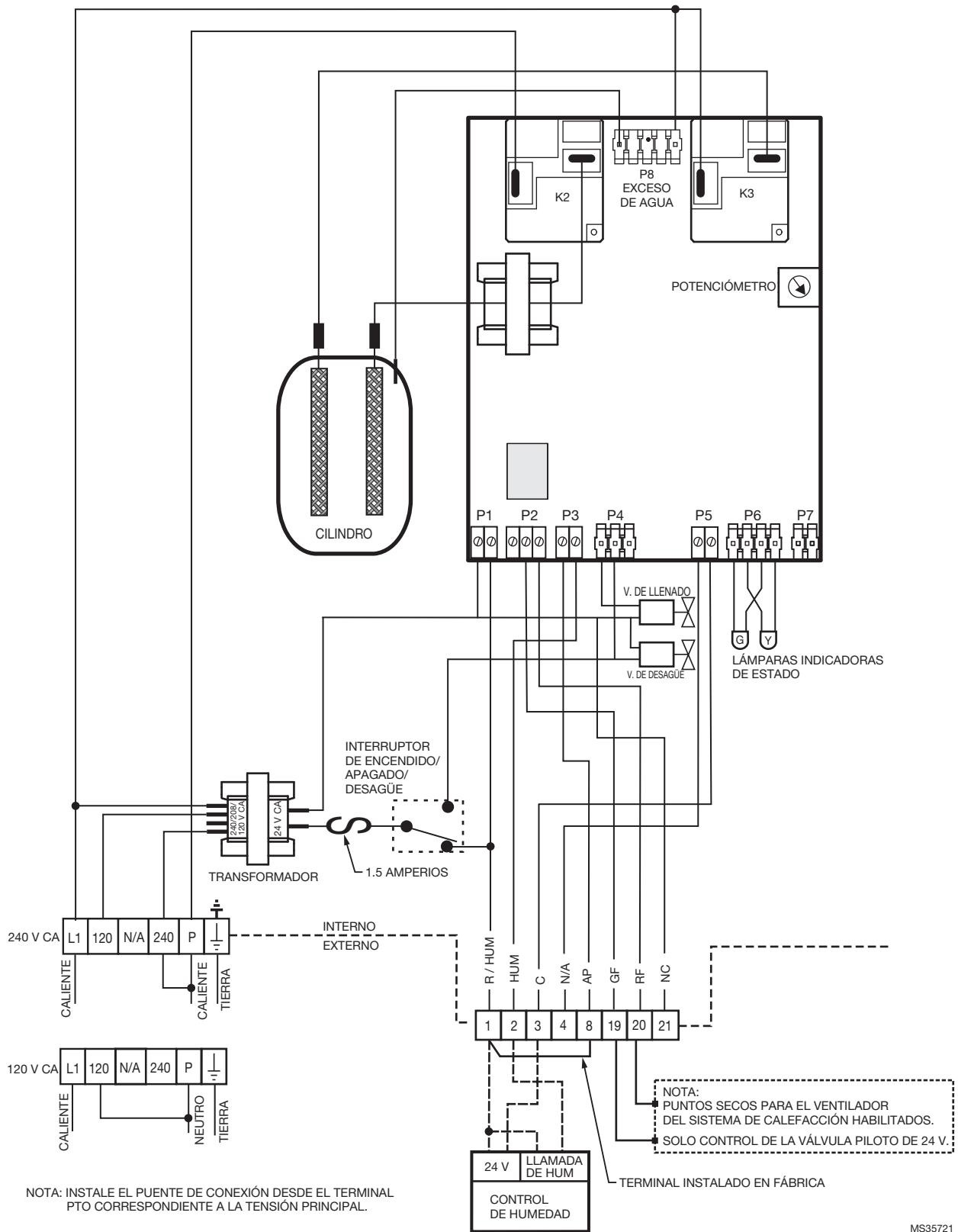
Fig. 12. Diagrama de cableado.
