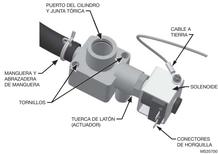
Fig. 3. Válvula de desagüe.
