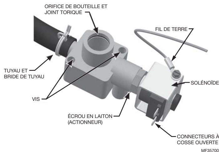
Fig. 2. Vanne de vidange.
