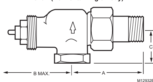
V2040A (Horizontal Angle Body)
