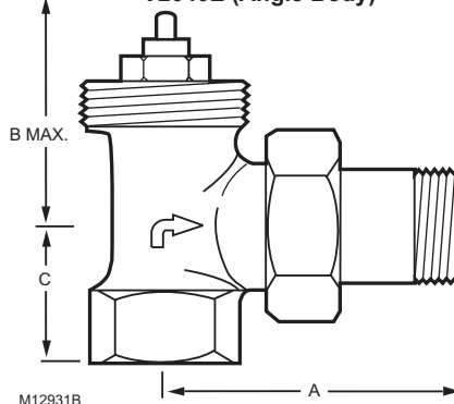
V2040E (Angle Body)
