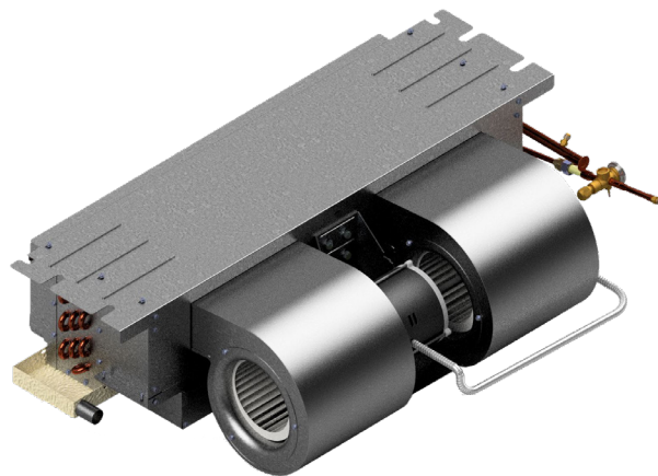
HX Fan Coil
