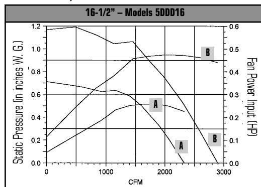
A = 5DDD168A, 870 RPM B = 5DDD16DB, 1140 RPM
