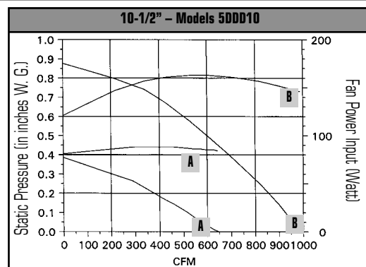
A = 5DDD106A, 1150 RPM B = 5DDD10AA, 1720 RPM
