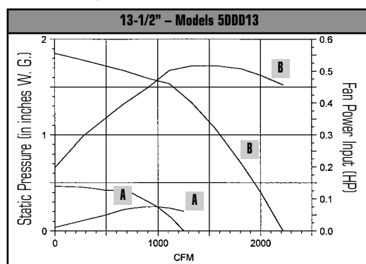
A = 5DDD138A, 870 RPM B = 5DDD13DB, 1680 RPM
