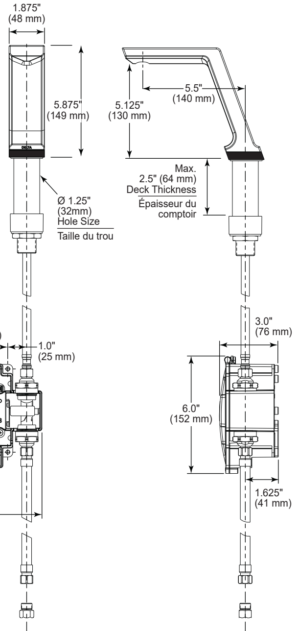
Single Hole Faucet with Black Spacer Robinet monotrou avec cale d'espacement noire
