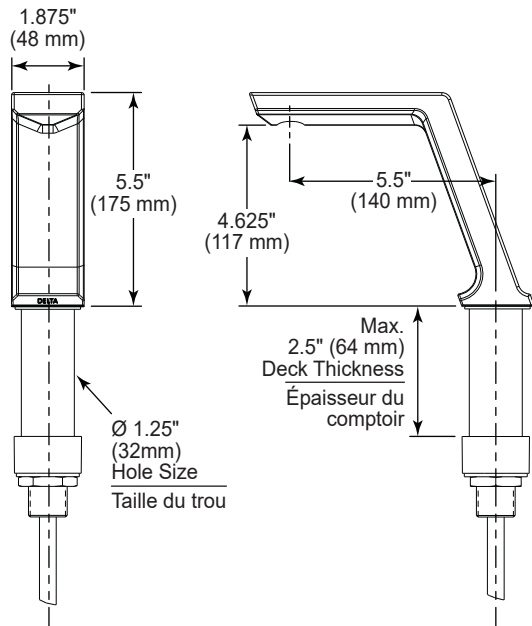
Single Hole Faucet without Black Spacer Robinet monotrou sans cale d'espacement noire
