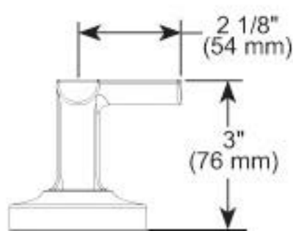
HX70406-▲ Cross Handle
