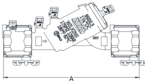
950XL3BFSS SHOWN
