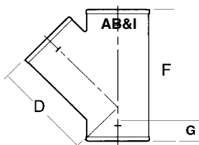
WYE (45°)
